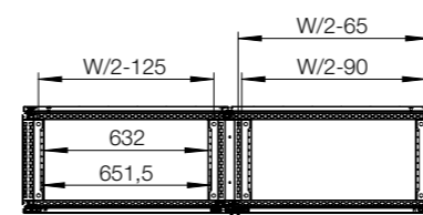
BEREICH C-C
