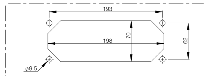
Ausschnitt
