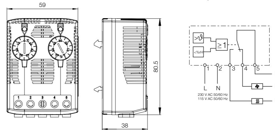
Frontansicht
