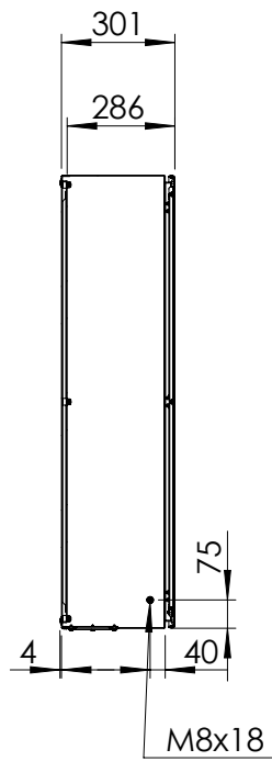
SECTION A-A
