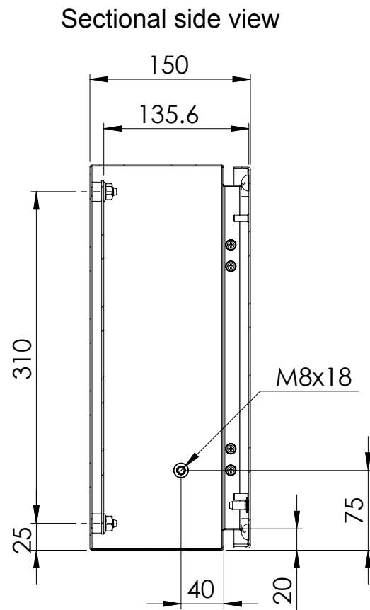
Section A-A
