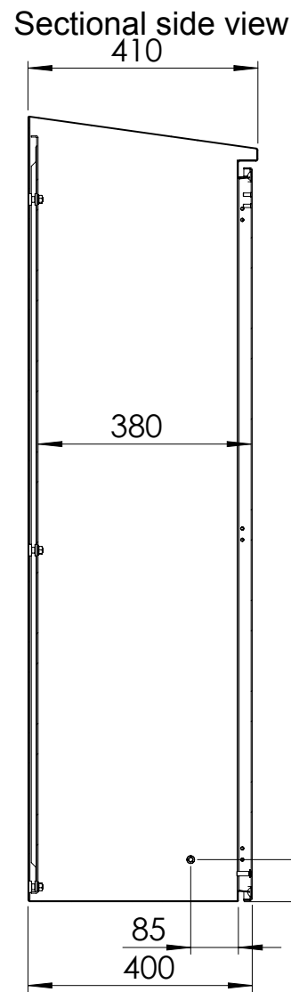
SECTION A-A
