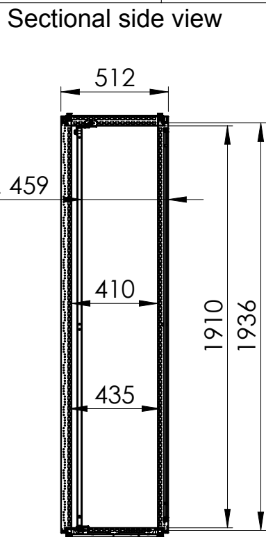
SECTION A-A
