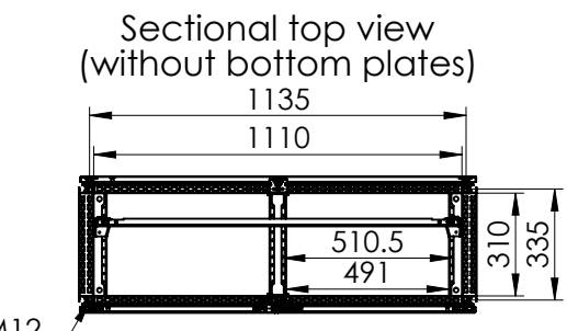
M12 SECTION B-B
