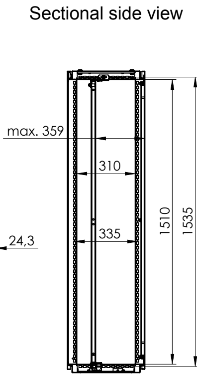
SECTION A-A
