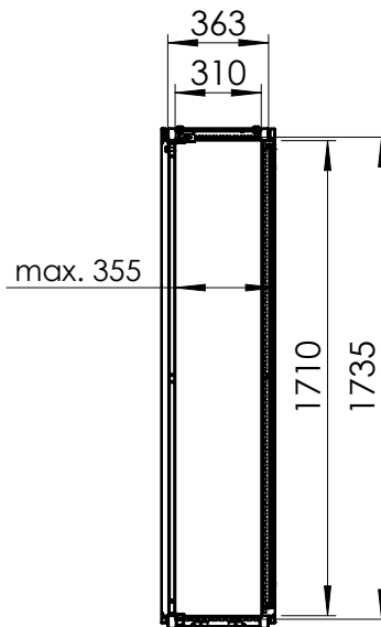
SECTION A-A SCALE 1 : 30
