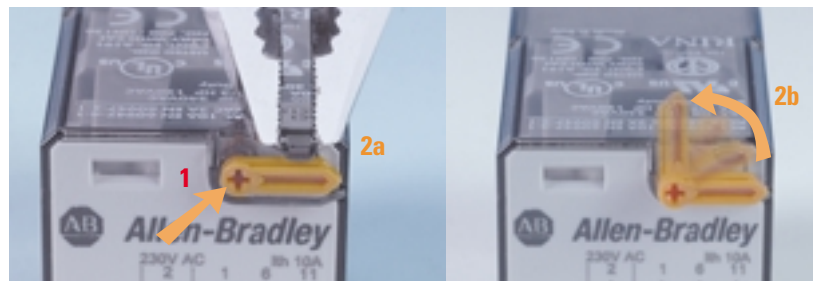
1 Prüftaste 2a Entfernen der Schutzlasche 2b Manuelle Betätigung der Kontakte
