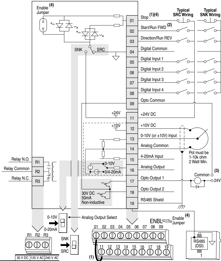
Steuerleitungsblockdiagramm
